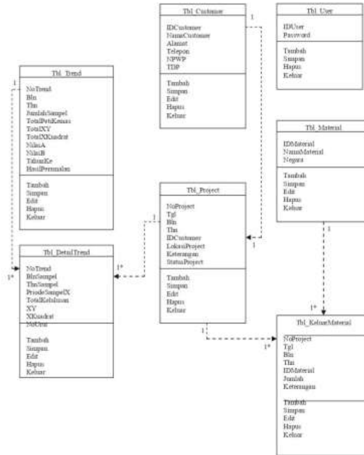
Gambar 6. Class Diagram Penerapan Statistical Parabolic Projection Untuk Kebutuhan Material Konstruksi PT. Andika Pratama Jaya Abadi Berbasis Web
