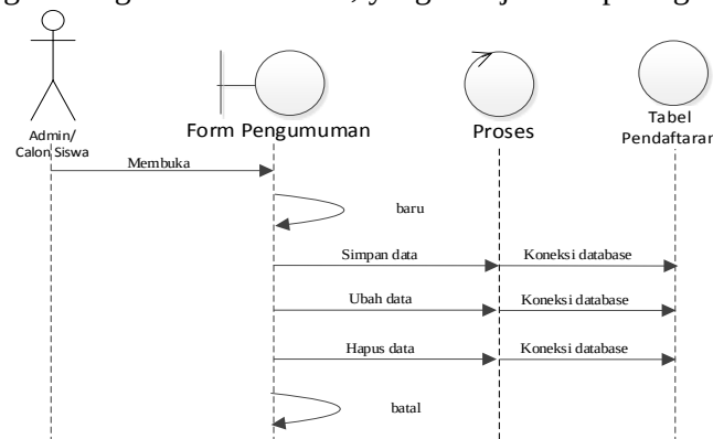
Gambar 17. Sequence Diagram Laporan Pengumuman
