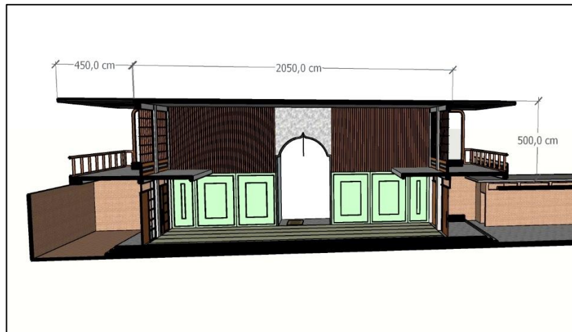
Gambar 13. Tampak Potongan B-B (Sumber : Muhammad Abi Nubli, 2023)
