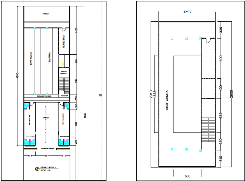
Gambar 3. Layout Lantai 1 dan lantai 2 (Sumber : Muhammad Abi Nubli, 2023)
