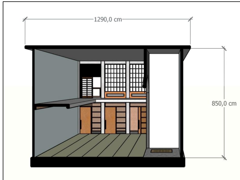
Gambar 12. Tampak Potongan A-A (Sumber : Muhammad Abi Nubli, 2023)
