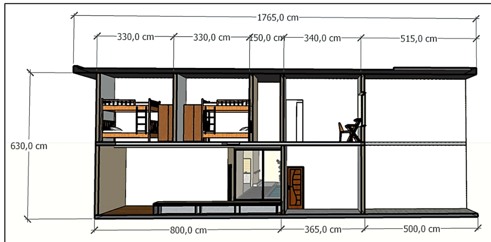
Gambar 17. Tampak Potongan A-A (Sumber : Suci Lestari, 2023)
