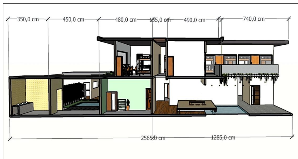
Gambar 18. Tampak Potongan B-B (Sumber : Suci Lestari, 2023)
